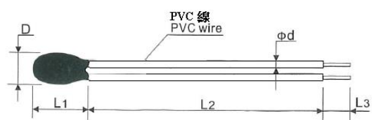
D型: 引線為PVC線 Model D: PVC wire
