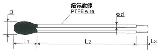
C型: 引線為鐵氟龍線 Model C: PTFE wire
